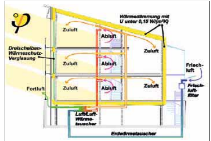
Schematischer Aufbau Passivhaus, Quelle: Wikipedia
